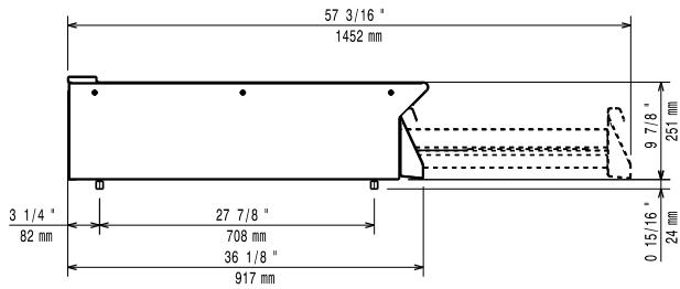
俯视
